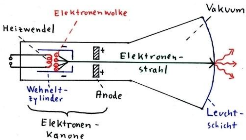
Abb 1: Prinzip der Braunschen Röhre
