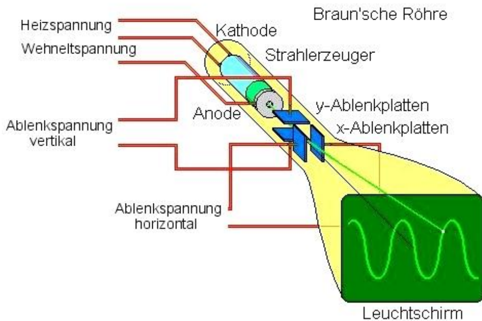
Abb 1: Prinzip der Braunschen Röhre
